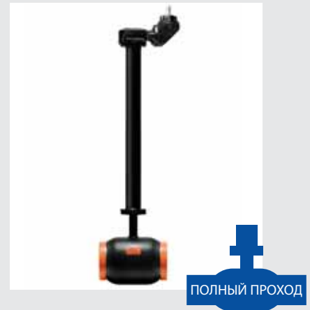
КШТ Серия 24, DN 350–1200, PN 2,5 МПа
